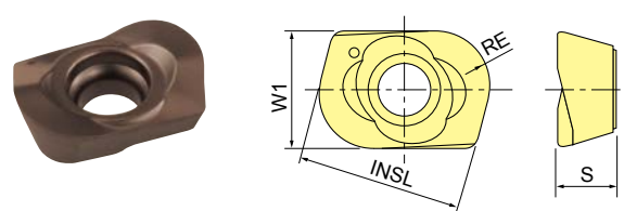
Fig-4 EDMT070220R(-T) コーナR2.0mmの低切込み高送り用インサート Insert with 2.0mm corner R for small-depth, high-feed-rate cutting (APMX=0.3mm)
